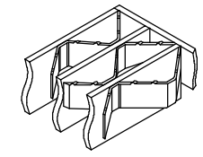
スベリ止め詳細図(N.T.S)
