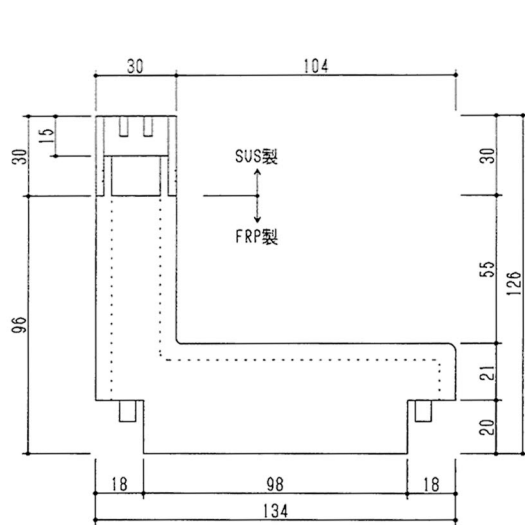
詳細図 S=1/2
