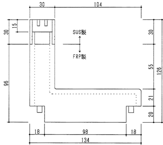
詳細図 S=1/2
