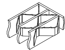
スベリ止め詳細図(N.T.S)
